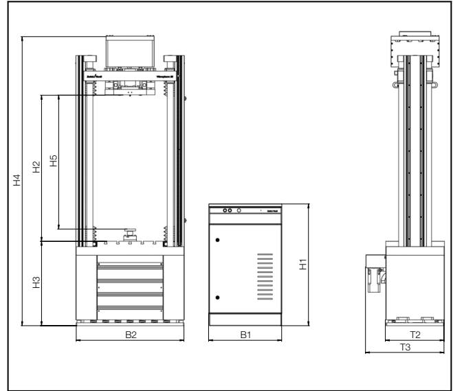
Zeichnung: Vibrophore 25
